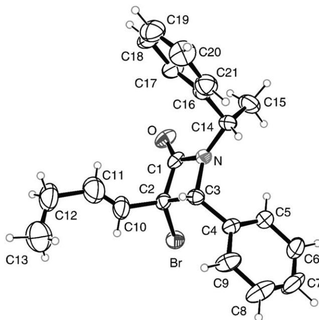
Figure 1. ORTEP diagram of 4e .
